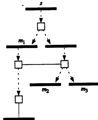
(d) truncated-broadcast delivery
