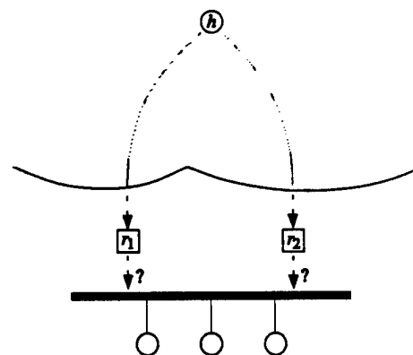
(d) reverse-path forwarding on multi-access links
